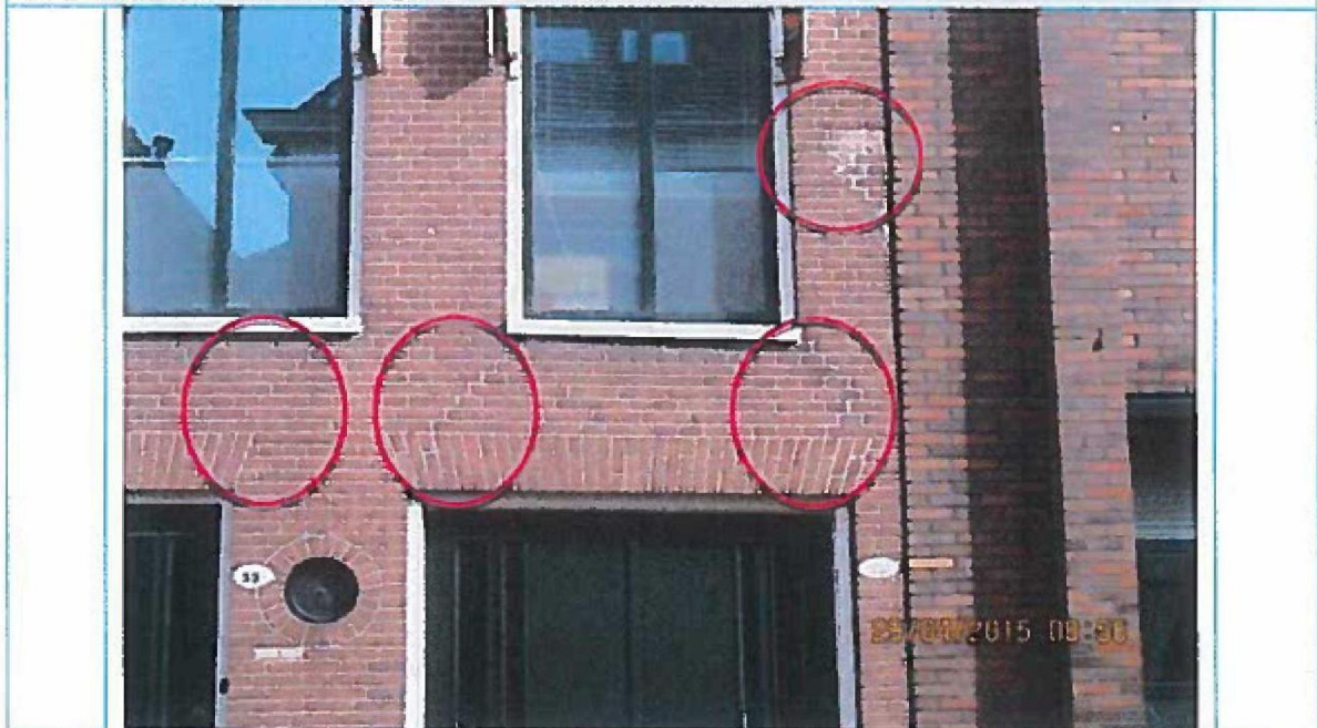
Foto 2. Reeds eerder hersteld voegwerk. Geen waarneembare schade.
