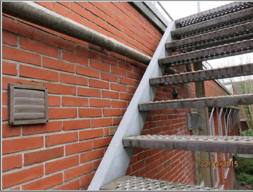
Schade 14, Horizontale scheuren en losse stenen (57784 22-4 (162))
