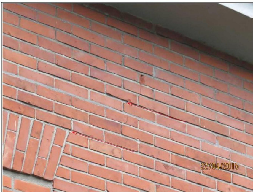
Schade 13, Verticale scheur door voegen en stenen (57784 22-4 (150))
