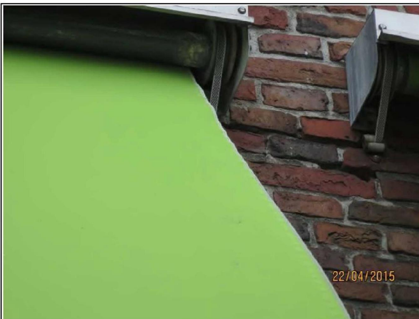
Schade 5, Horizontale scheur in de voeg. (57784 22-4 (93))
