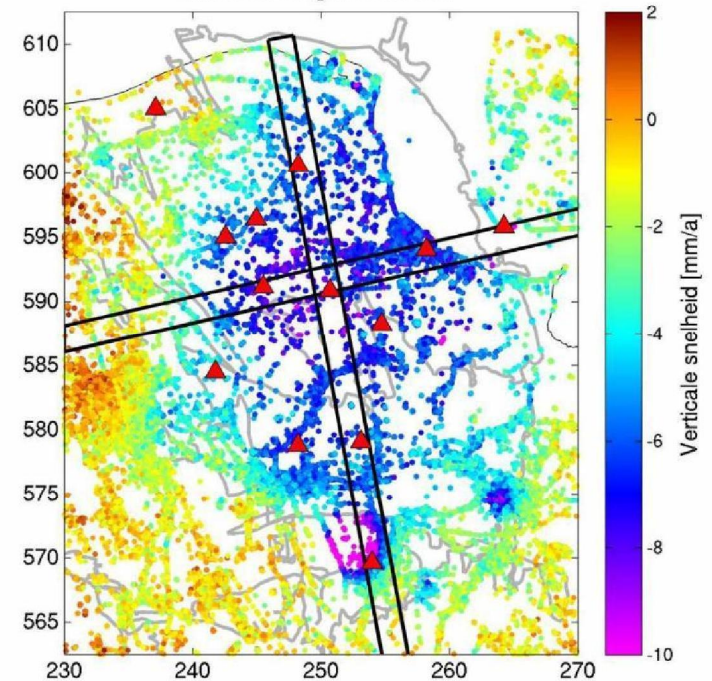
InSAR Groningen 2009-2014
