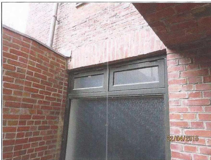
Schade 8, Scheurvorming in metselwerk (57784 22-4 (108))
