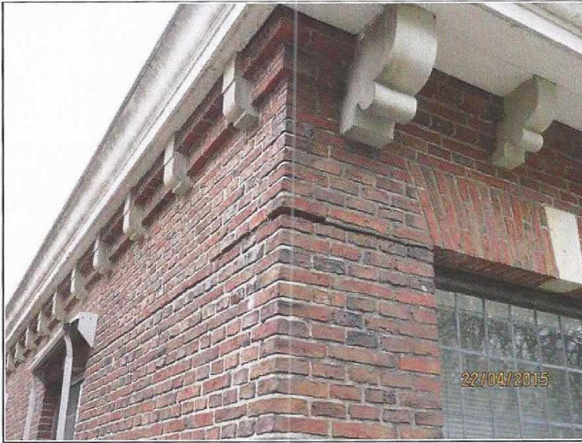
Schade 1, Horizontale scheur in de voeg. (57784 22-4 (48))
