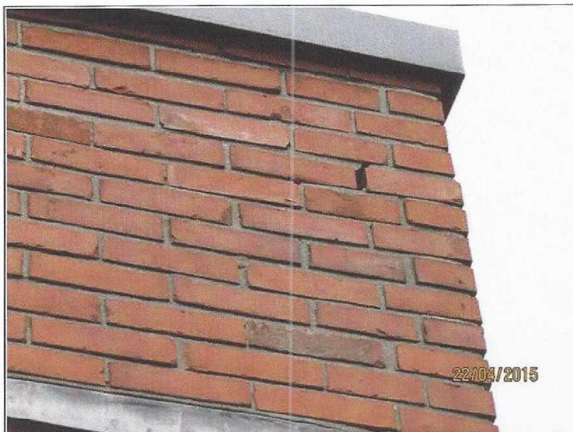
Schade 12, Horizontale scheuren en losse stenen (57784 22-4 (137))
