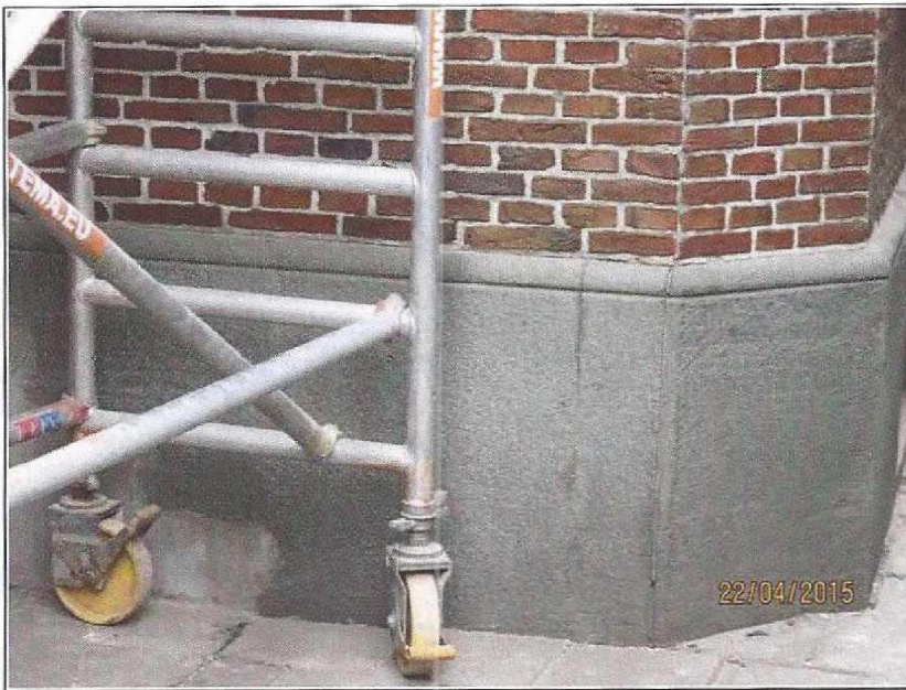
Schade 4, Verticale scheur in natuursteen plint (57784 22-4 (82))
