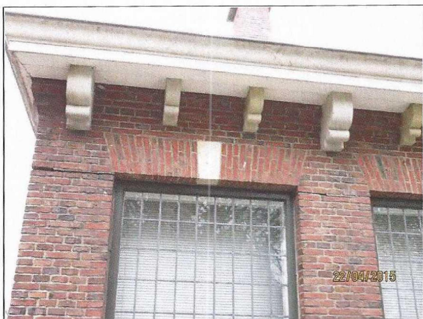
Schade 1, Horizontale scheur in de voeg. (57784 22-4 (37))
