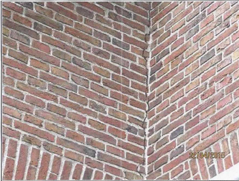
Schade 10, Verticale scheur in hoek aansluiting (57784 22-4 (121))
