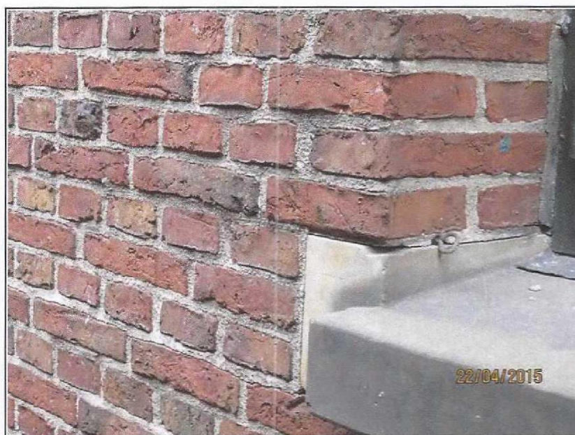
Schade 3, Verticale en horizontale scheuren (57784 22-4 (74))
