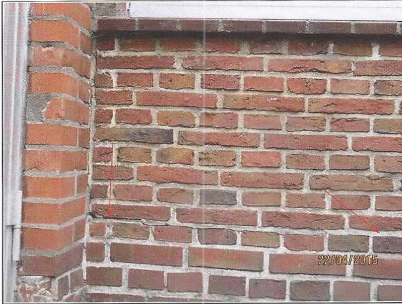
Schade 11, Diverse scheuren in voeg en stenen. (57784 22-4 (130))
