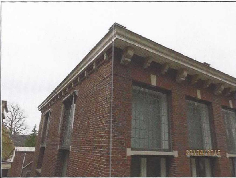
Schade 1, Horizontale scheur in de voeg. (57784 22-4 (45))
