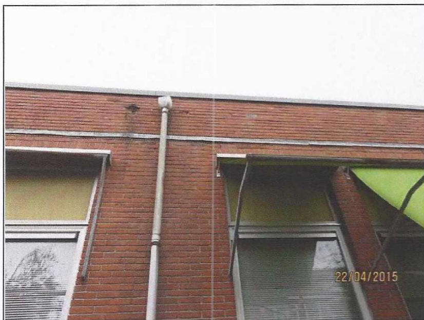
Schade 12, Horizontale scheuren en losse stenen (57784 22-4 (138))
