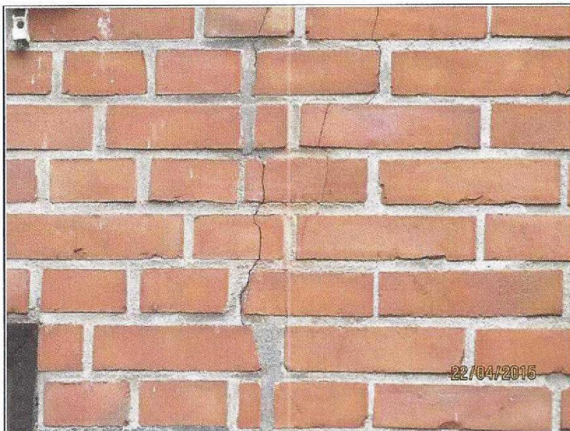
Schade 15, Verticale scheur door stenen en voegen (57784 22-4 (160))
