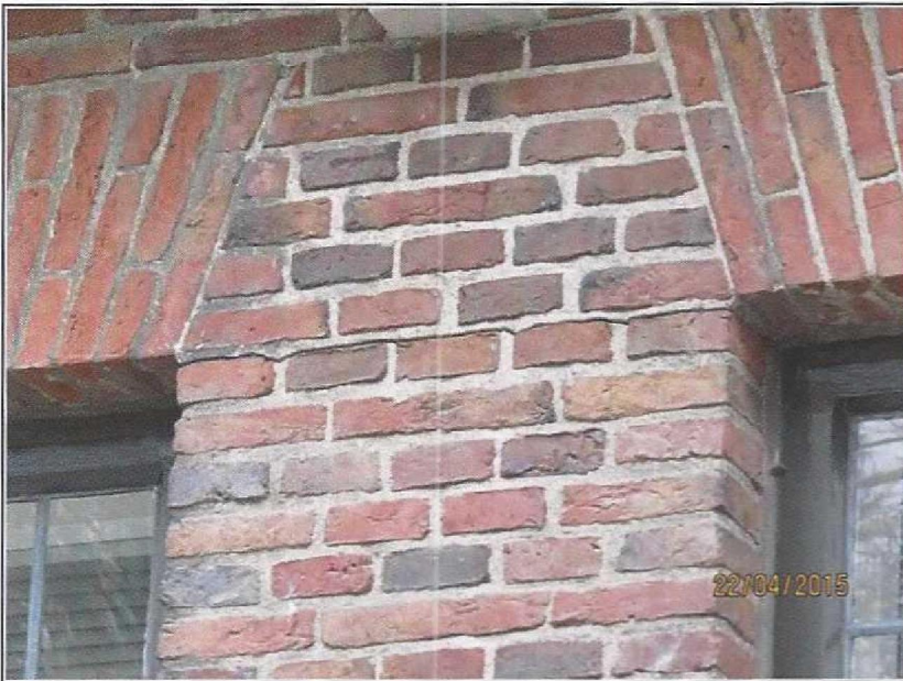
Schade 1, Horizontale scheur in de voeg. (57784 22-4 (35))
