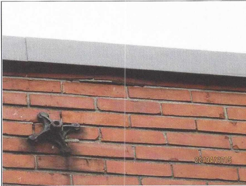
Schade 12, Horizontale scheuren en losse stenen (57784 22-4 (141))
