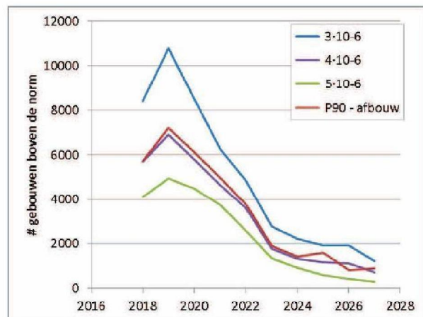
Figuur II-2: Weergave van het aantal gebouwen dat in aanmerking komt voor versterking op basis van enkele signaleringswaarden: 3 \cdot 10^{-6} per jaar, 4 \cdot 10^{-6} per jaar en 5 \cdot 10^{-6} per jaar.
