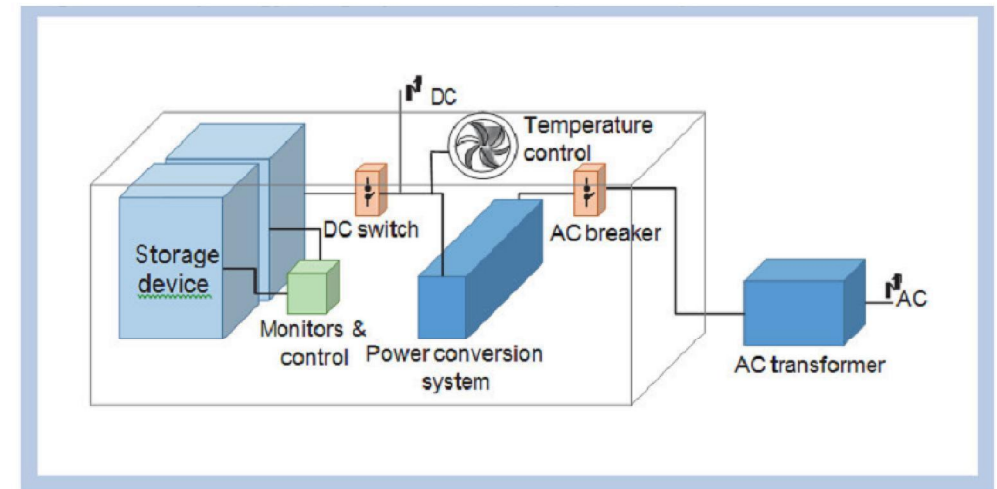
Figuur: Batterij opslag systeem en de primaire componenten
