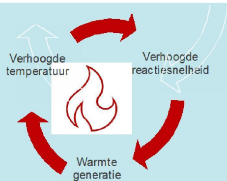
Figuur: Feedbackmechanisme thermal runaway
