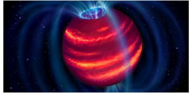
Artist impression van Elegast. De blauwe lijnen geven de magnetische veldlijnen weer. Geladen deeltjes die langs deze lijnen bewegen, zenden radiogolven uit die LOFAR detecteert. (Credit: ASTRON/Daniëlle Futselaar)
