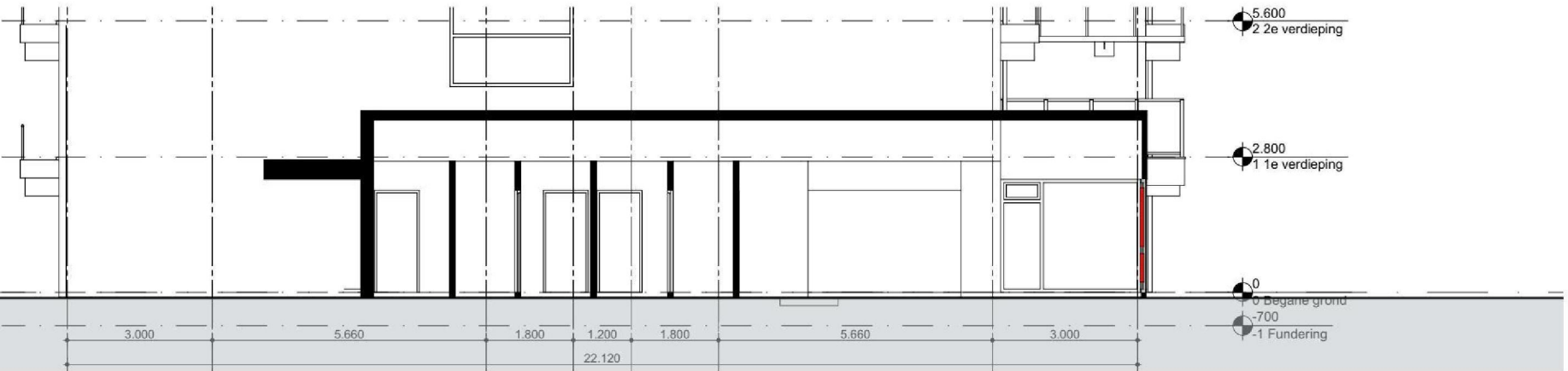
doorsnede B - B
