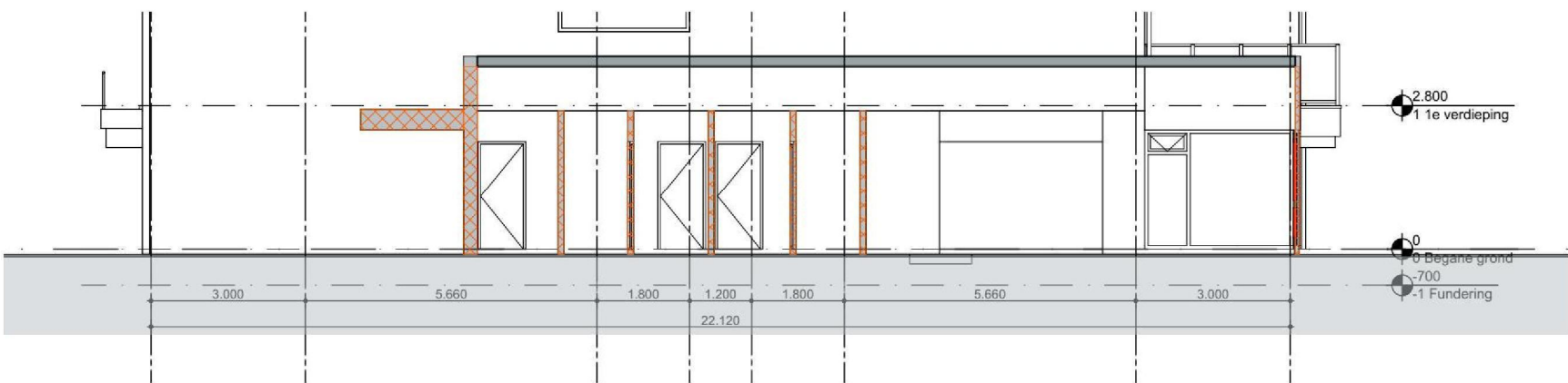
Doorsnede B - B
