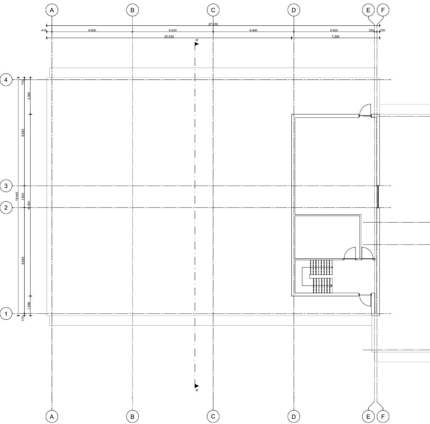
11e verdieping
